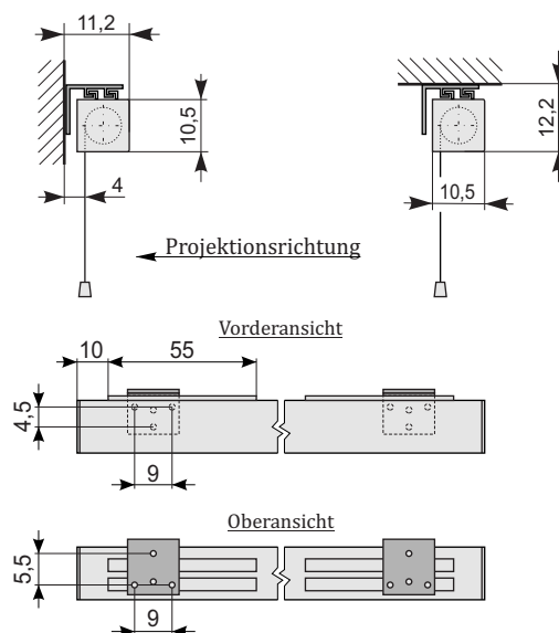
Wandschalter
